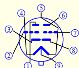
12AX7管脚图
