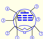
EL34管脚图
