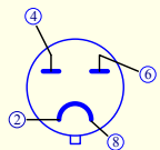
5U4/5Z3P管脚图
