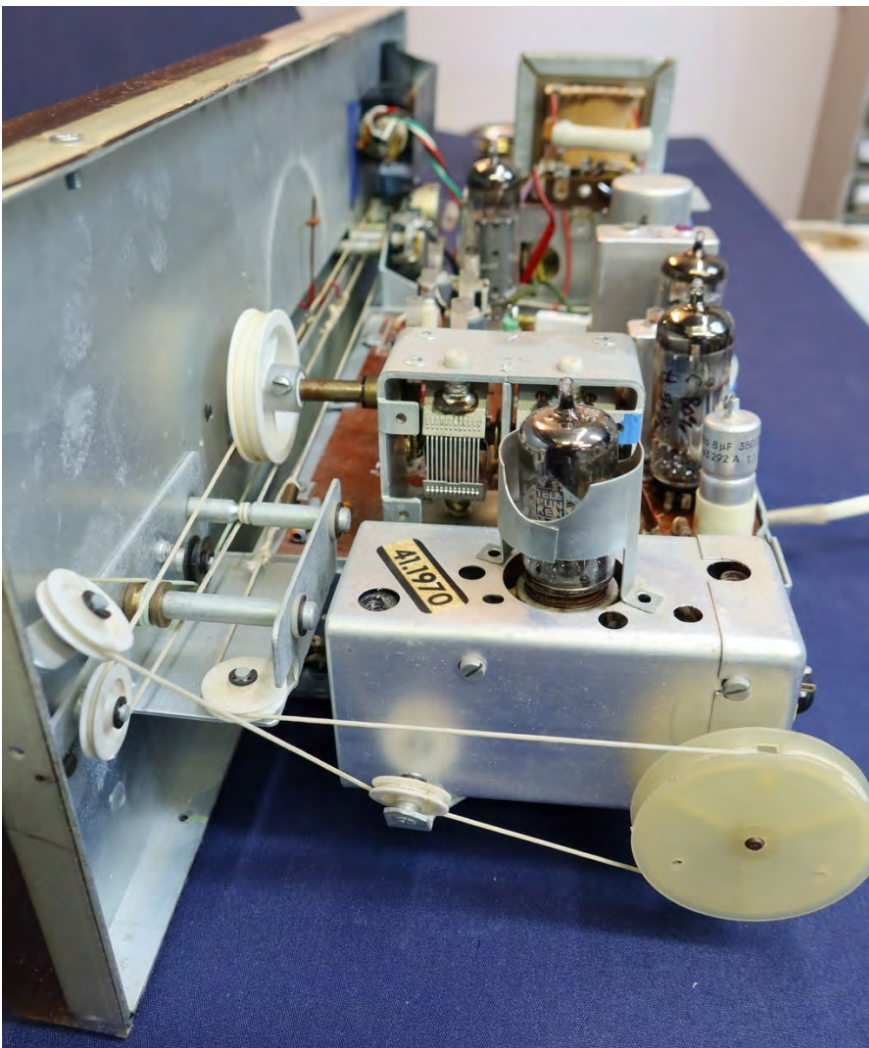
Futura (1) Ulapurkki ja narutus. Futura (2) alla
