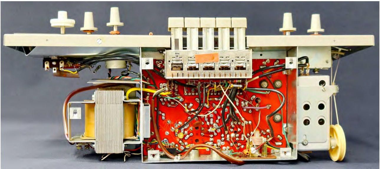
Futura Koneisto alta.
