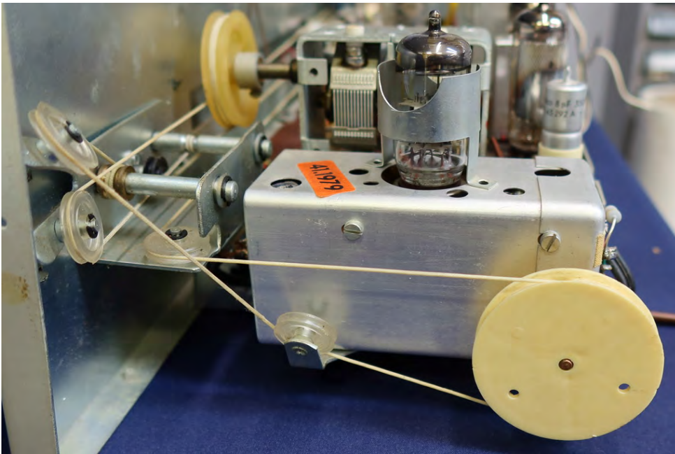
Futura (1) Ulapurkki ja narutus. Futura (2) alla
